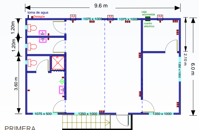
PRIMERA PLANTA
