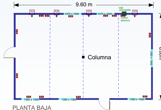
PLANTA BAJA
