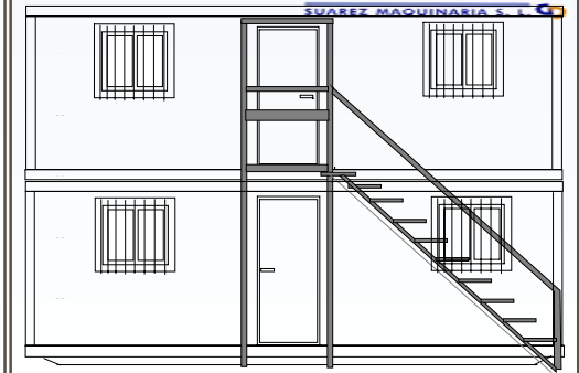
2 CASETAS G8AD APILADAS
