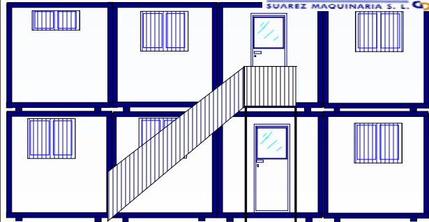
ALZADO FRONTAL
