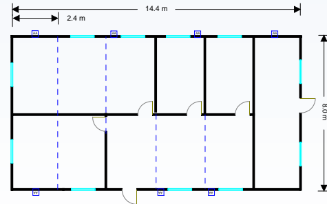
CONJUNTO MODULAR 6 M8AE
