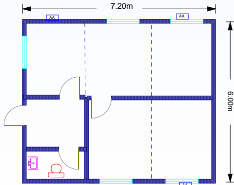
CONJUNTO MODULAR 3 M6AE
